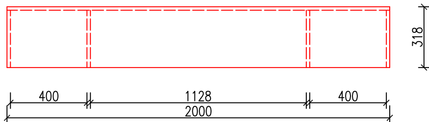
PŮDORYS
