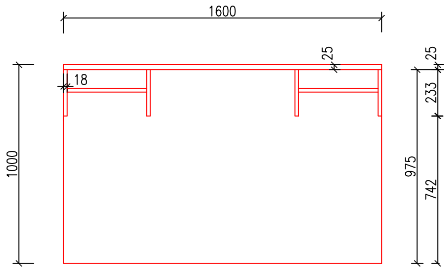
NÁRYS
